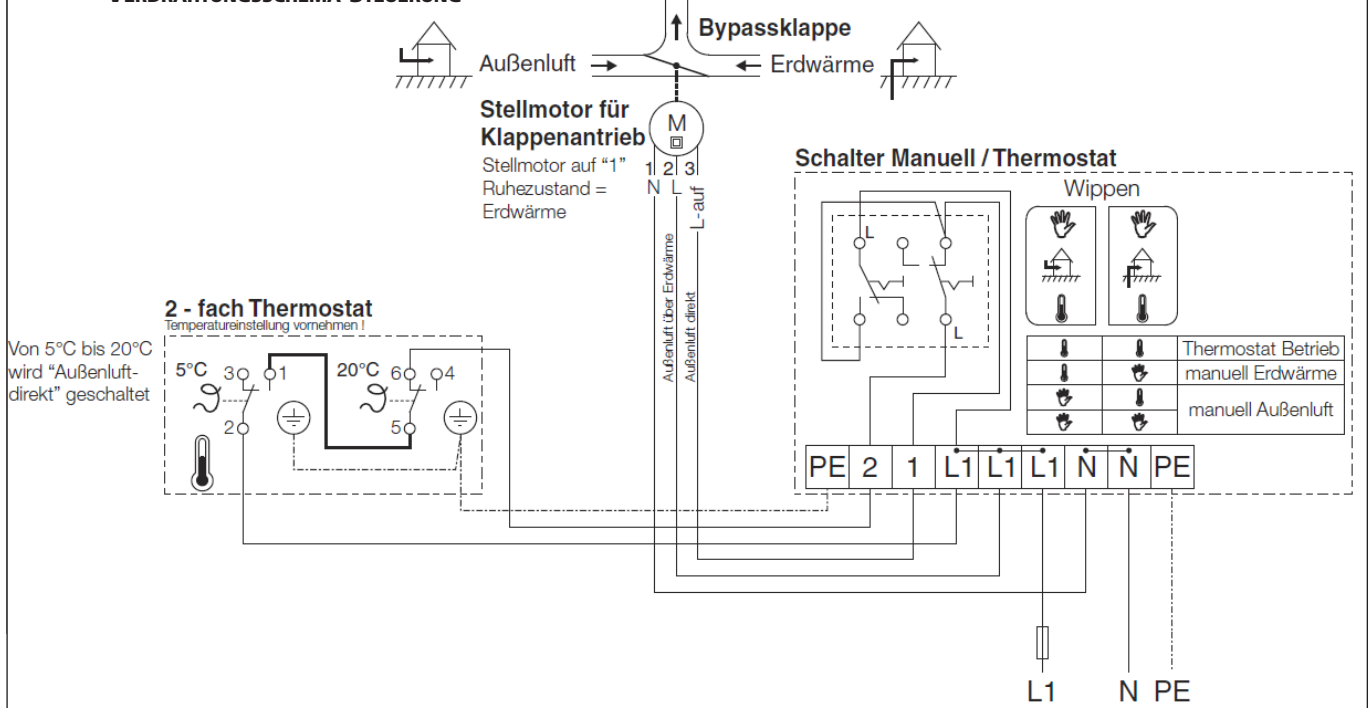
Abb. 3 VERDRÄHTUNGSSCHEMA STEUERUNG
